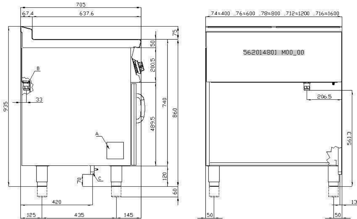
FIG. 1 TP..-7..G
